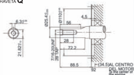
OHV240 OHV270 CHAVETA Q
