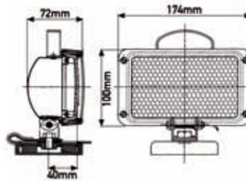
RMFTR712 H3 12V 55W
