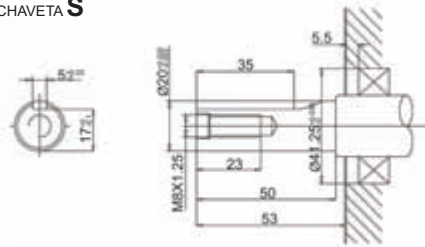
OHV200 CHAVETA S
