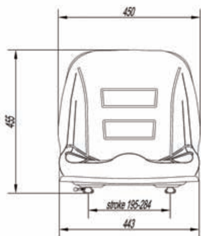
RM700B diseño M99
