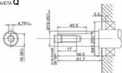
OHV160 CHAVETA Q
