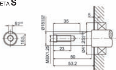
OHV120 CHAVETA S
