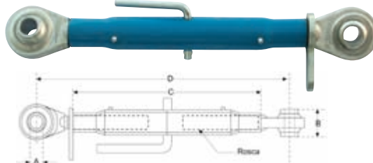
Tercer punto reforzado Top link assembly, metric-heavy duty 62TLH0226 - 62TLR0253
