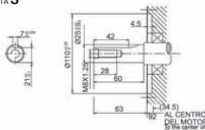
OHV240 OHV270 CHAVETA S
