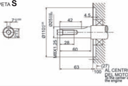
OHV340 OHV390 CHAVETA S
