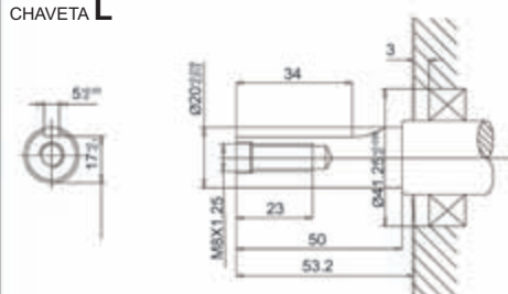
OHV160 CHAVETA L
